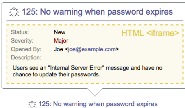
Fig. 2 Preview iframe
